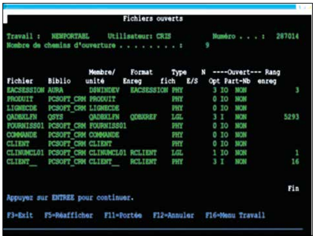
Visualisation des I/O sur l'AS/400. Le buffer d'I/O est paramétrable pour chacun des fichiers. Il vous permet d'optimiser les performances selon votre besoin.
